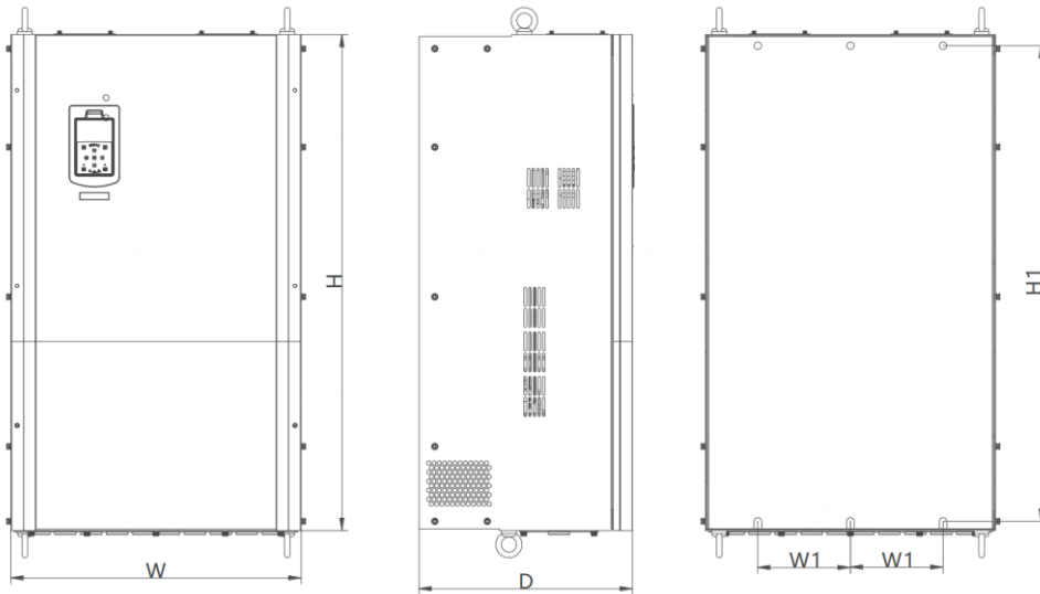
图 5-4 NVF3G-75QZ ~ NVF3G-132QZ 外形与安装尺寸图
