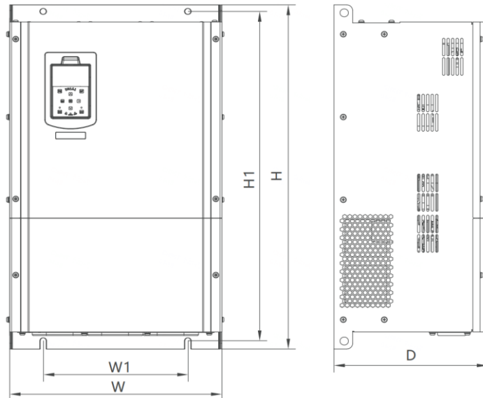
图 5-2 NVF3G-15QZ ~ NVF3G-45QZ 外形与安装尺寸图
