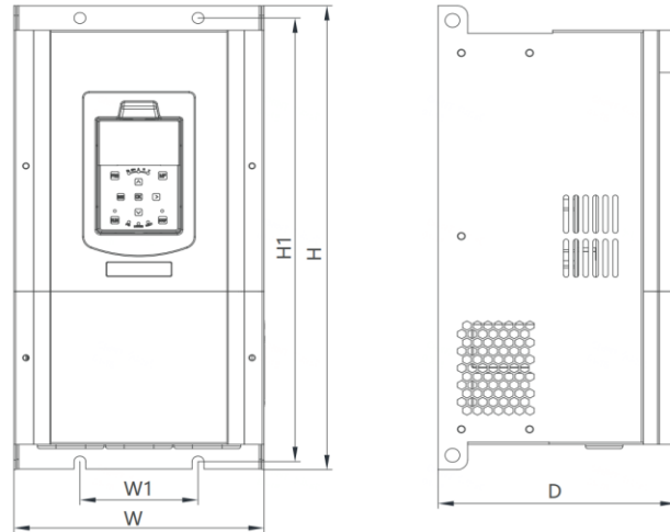
图 5-2 NVF3G-15QZ ~ NVF3G-45QZ 外形与安装尺寸图
