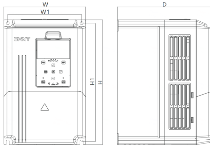
图 5-1 NVF3G-1.5QZ ~ NVF3G-11QZ 外形与安装尺寸图
